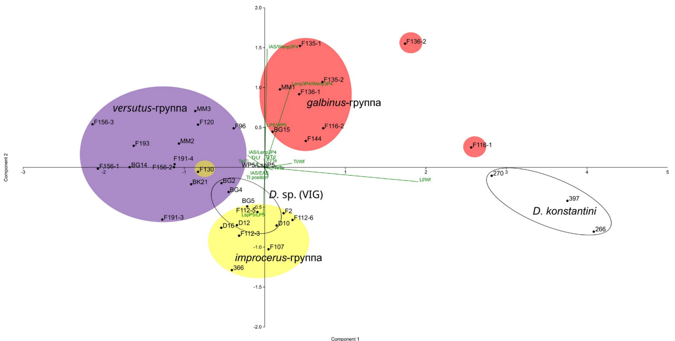
Рис.4. Результаты анализа главных компонент, примененного к байкальским Diacyclops на основе морфометрических индексов. Число означает номер особи. Зеленые стрелки показывают индексы и их вклад в первые две главные компоненты. Цвета овалов соответствуют цветам групп, отмеченных на филогенетических деревьях.
